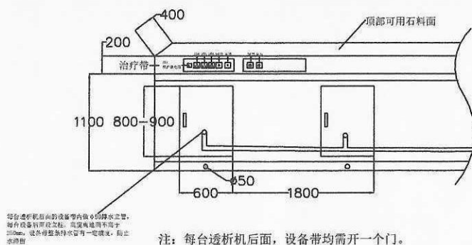
设备带示意图
